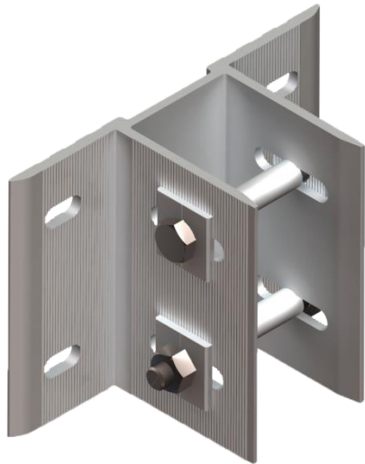
Кронштейн 80x120 01744
